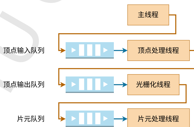
图 1.2: 光栅化渲染管线的流水结构
